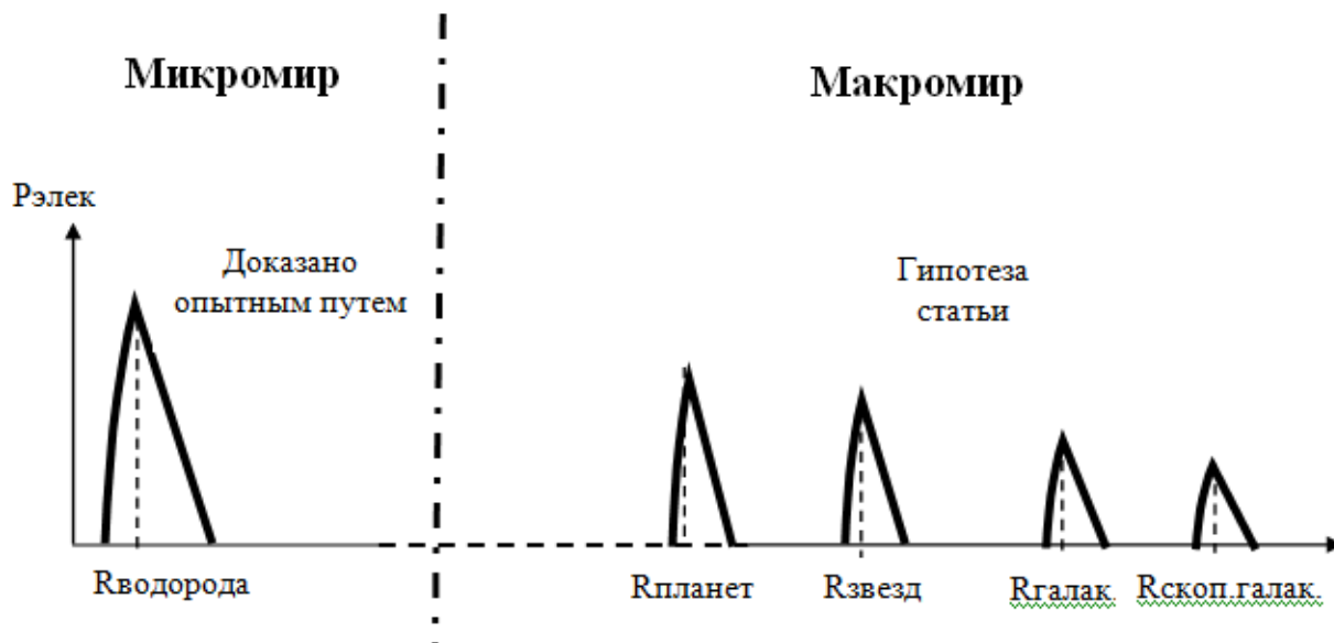
Рисунок 3 – График возможного радиального распределения вероятности для 1s-электрона атома водорода в микро и макро мирах
