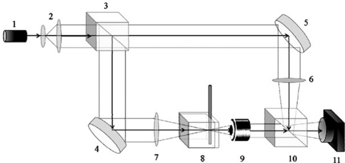
Рисунок 2 – Схема цифрового голографического микроскопа для исследования микросред: 1 лазер; 2 - коллиматор; 3, 10-светоделительные кубики; 4, 5 зеркала; 6, 7 линзы; 8 кювета с исследуемым оптоволокном; 9 - микрообъектив; 11 цифровая фотокамера.
