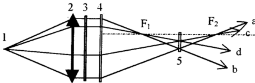
Рисунок 1 – Схема регистрации некогерентных голограмм.
