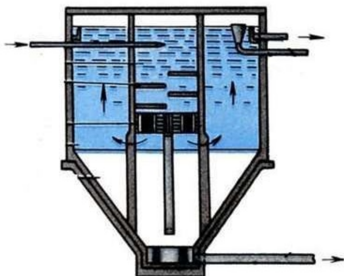
Fig. 1. Tank-sump
